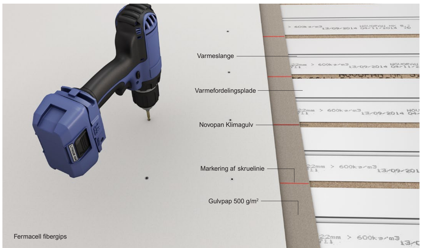
Figur 1 Novopan Klimagulv 22 og 25 mm forstærket med Fermacell fibergipsplader som mellemlag under gulvbelægning, se side 2.
